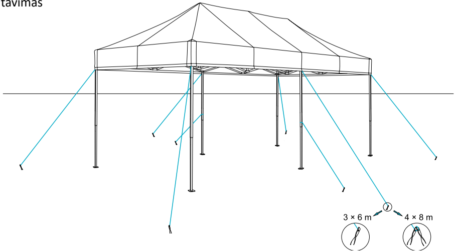
Lentelė nr.2. Palapinių rišimo būdai su nestandartinėmis konstrukcijomis
