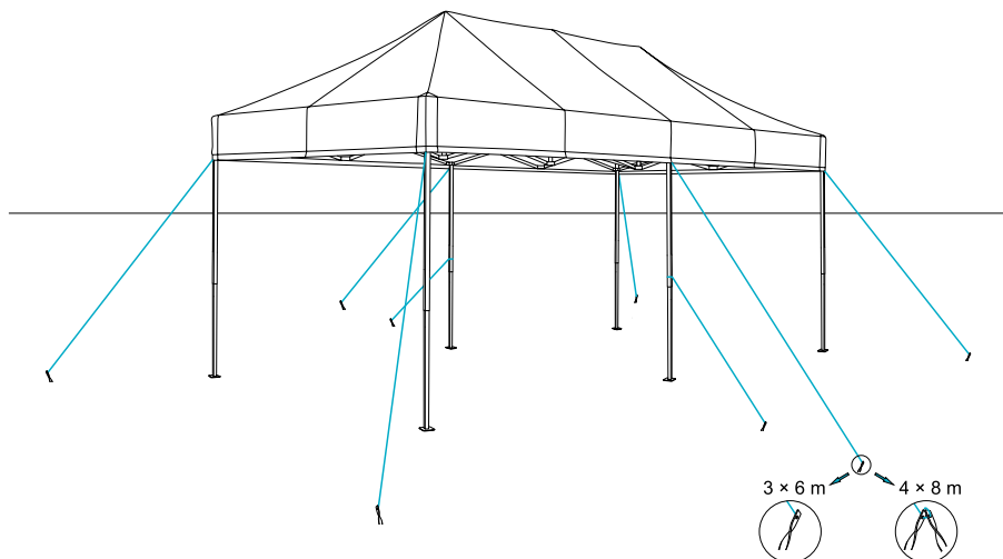
Tabulka 2. Způsoby kotvení nůžkového stanu na atypických konstrukcích
